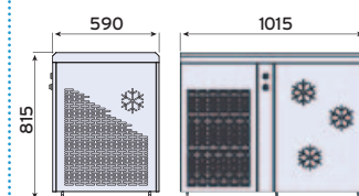
FIM 400
